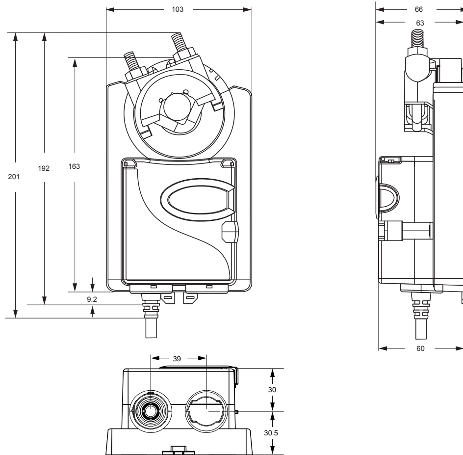
图8: 尺寸图
