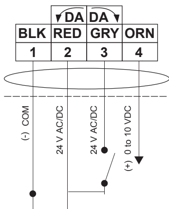
图2: 开关控制
