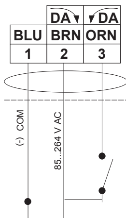
图6: 开关控制
